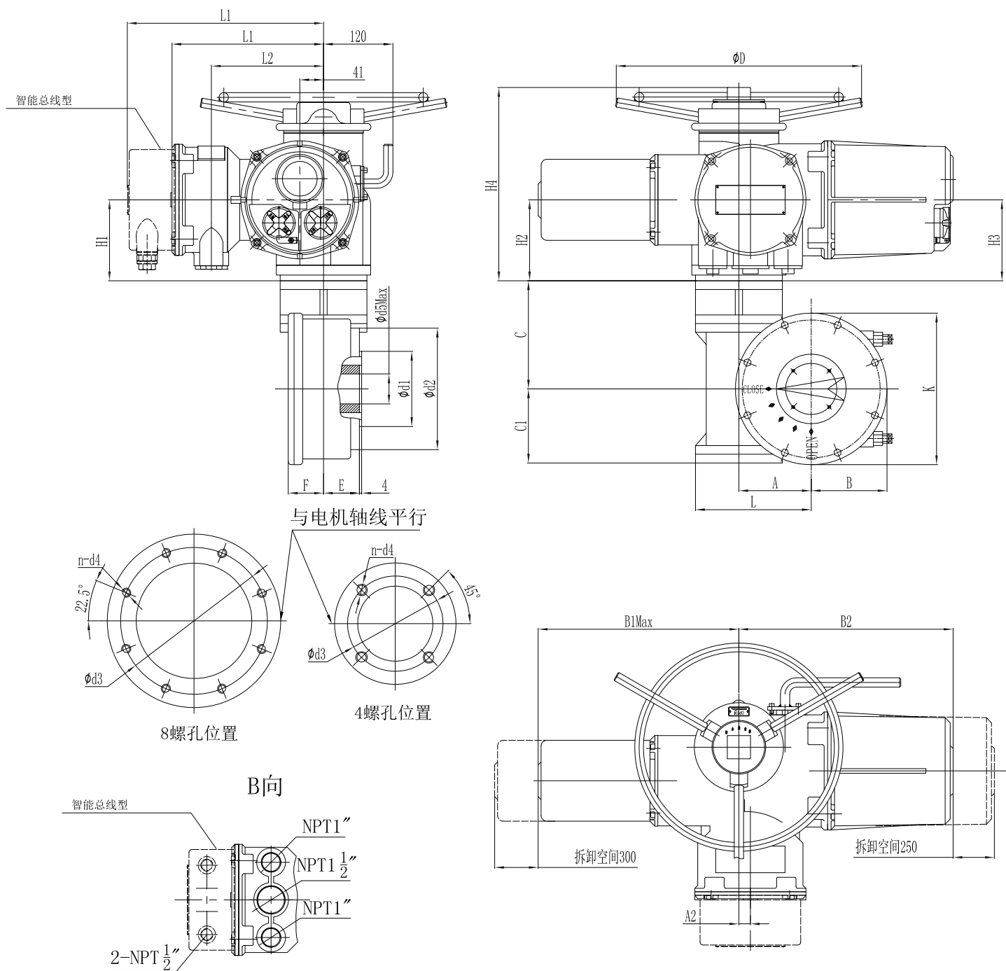
IMC15~60带HJBC系列外形及连接尺寸
